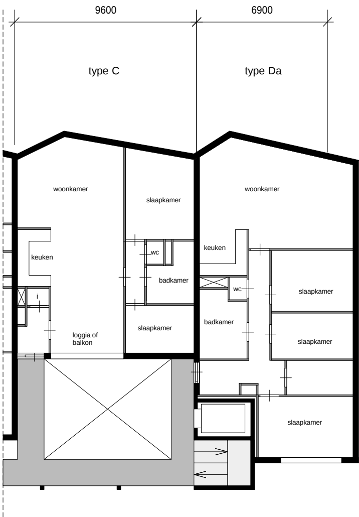
laag 3 1:200
