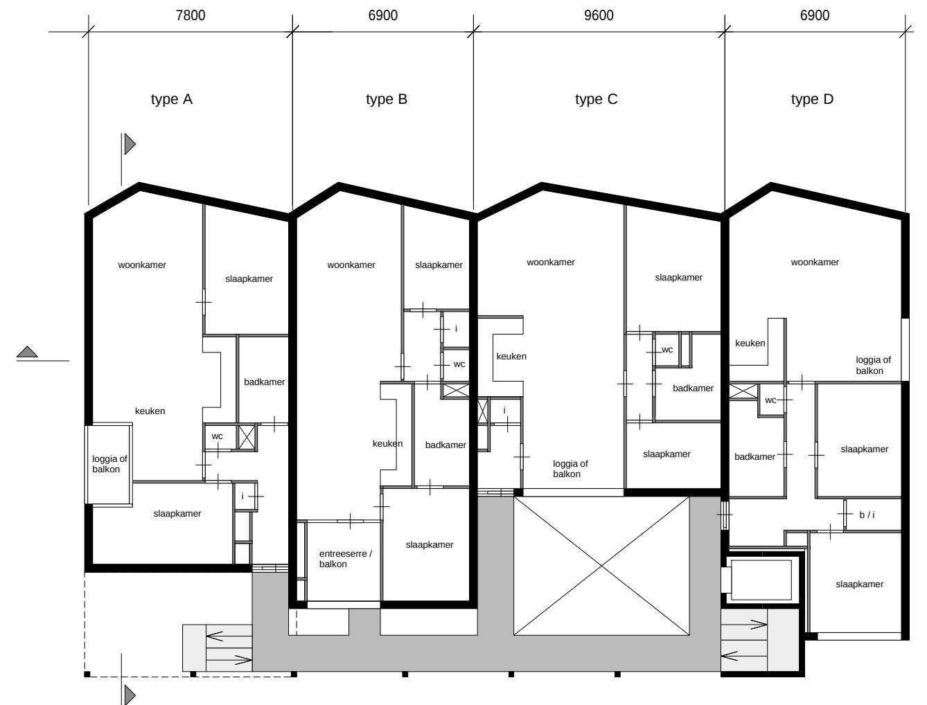
laag 2 1:200 noordgevel 1:200
