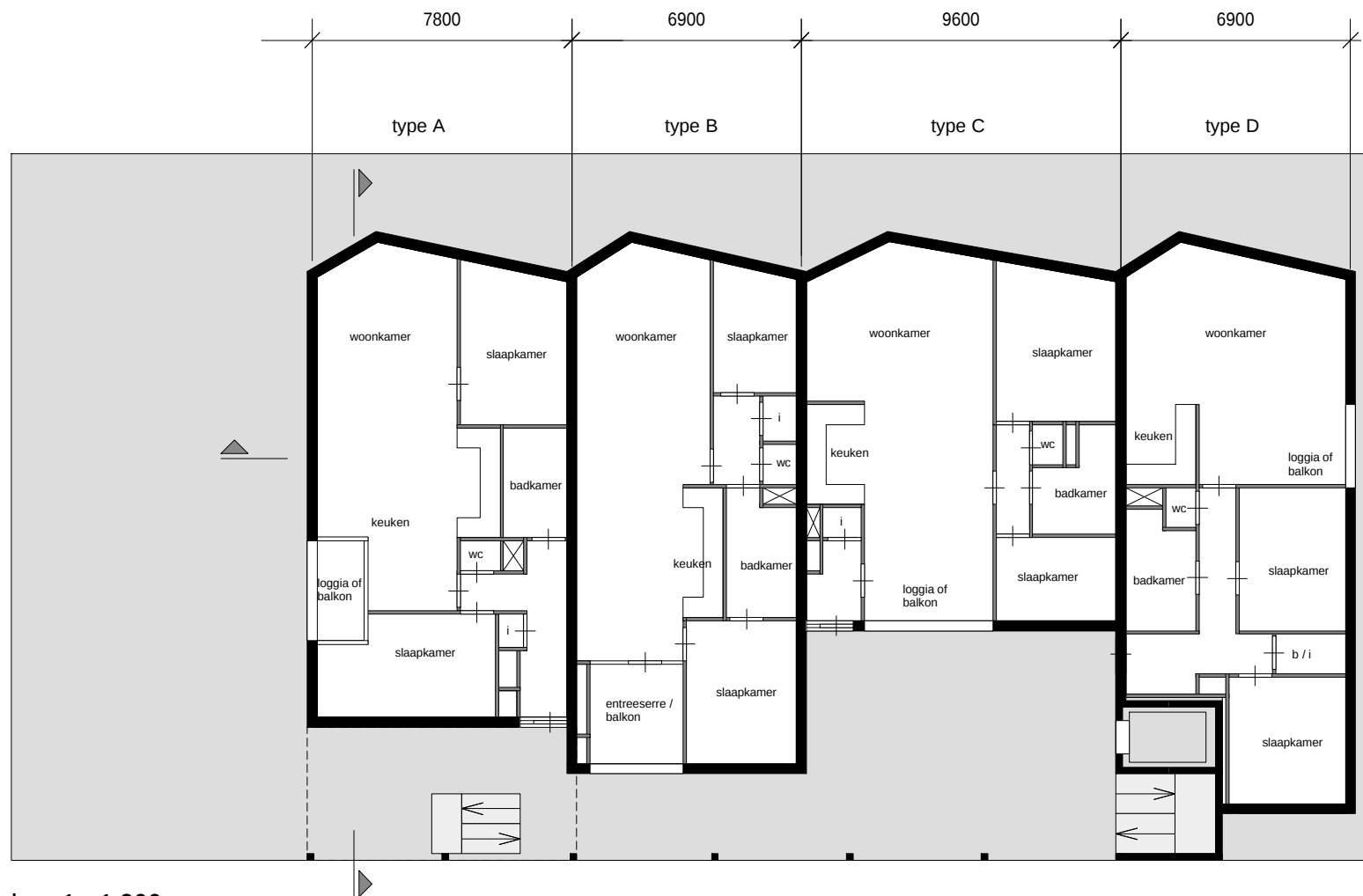
laag 1 1:200 westgevel 1:200
